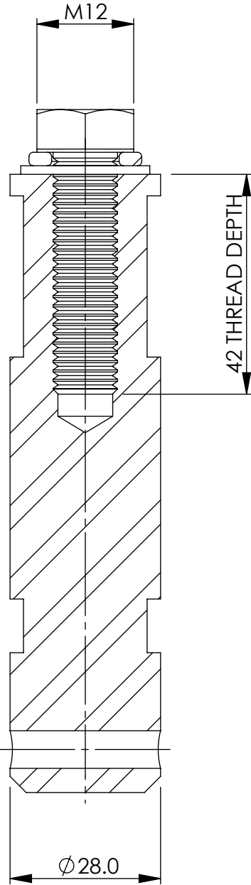
SECTION A-A
