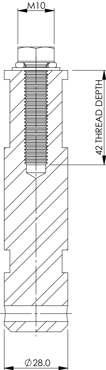
SECTION A-A
